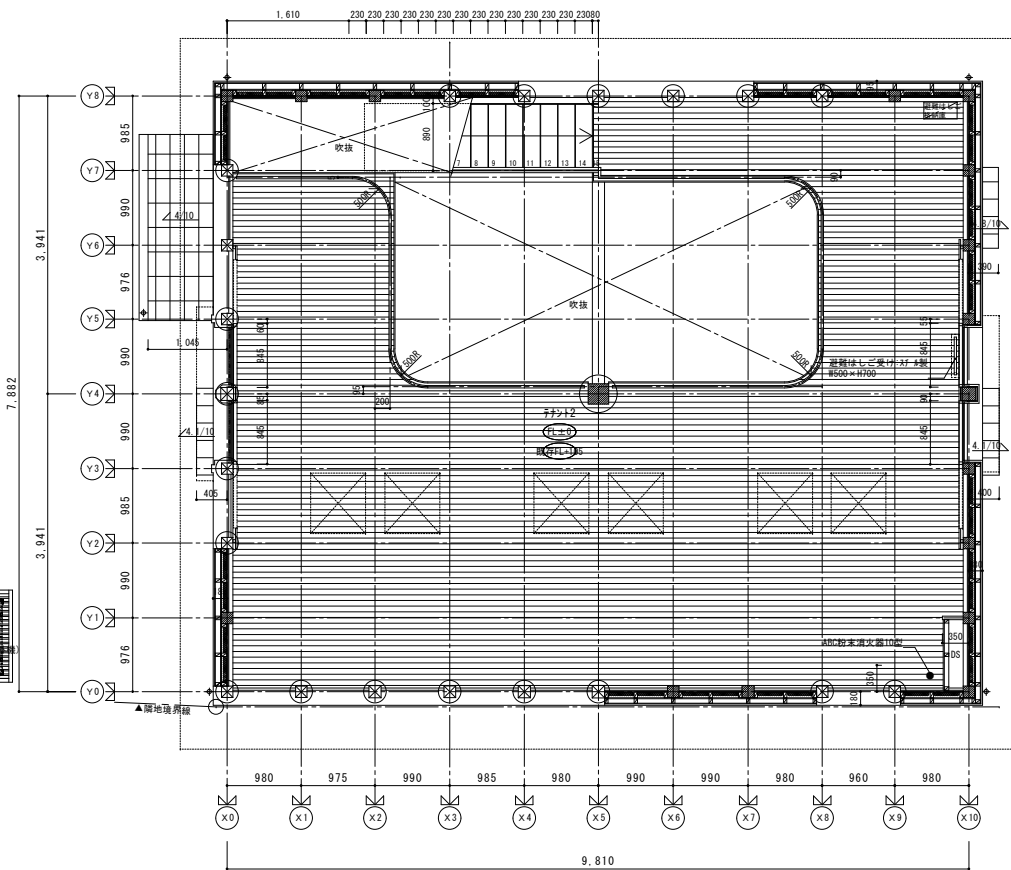
2階平面詳細図
