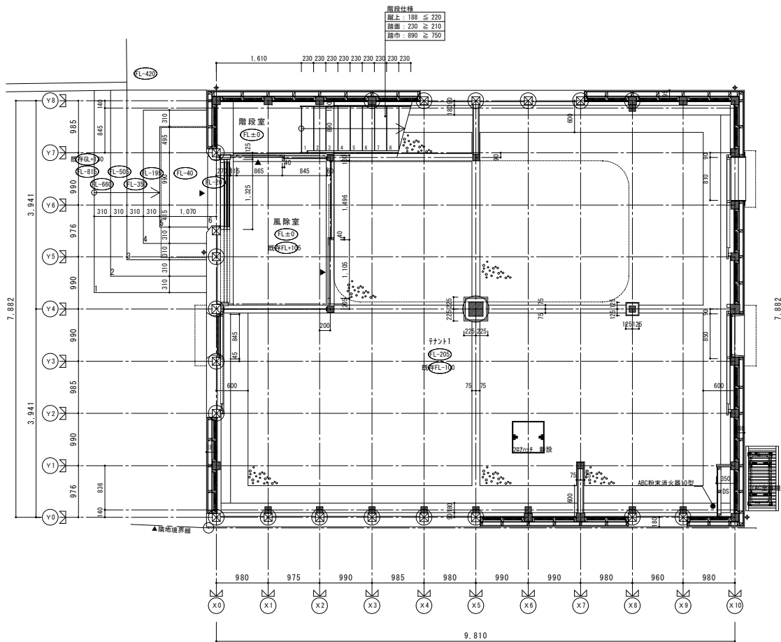
1階平面詳細図
