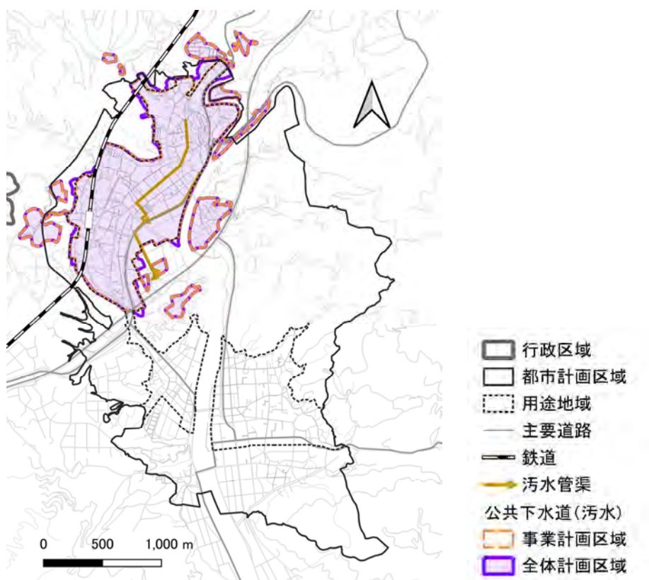
公共下水道（污水） 位置図
