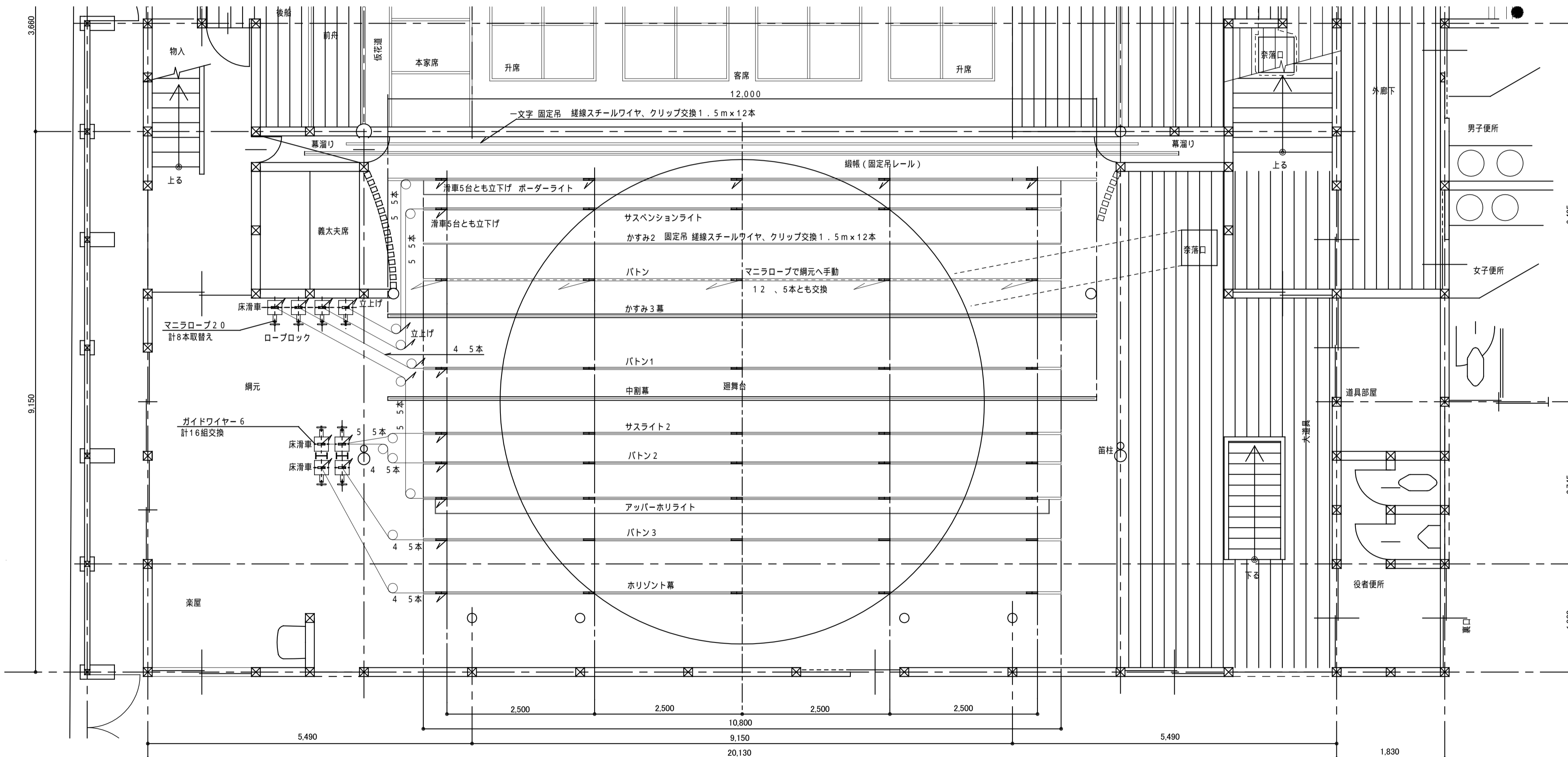
平面図 S=1:50
