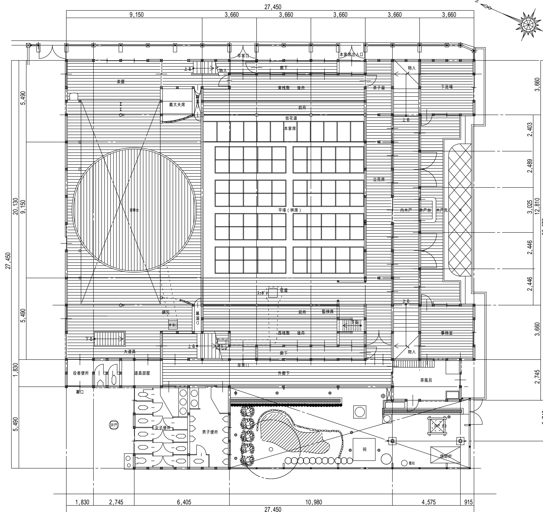
1階平面図 S=1:150
